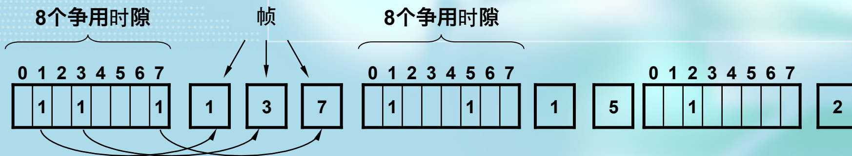
Tnbm P259 Fig. 4 – 6 基本位图协议
