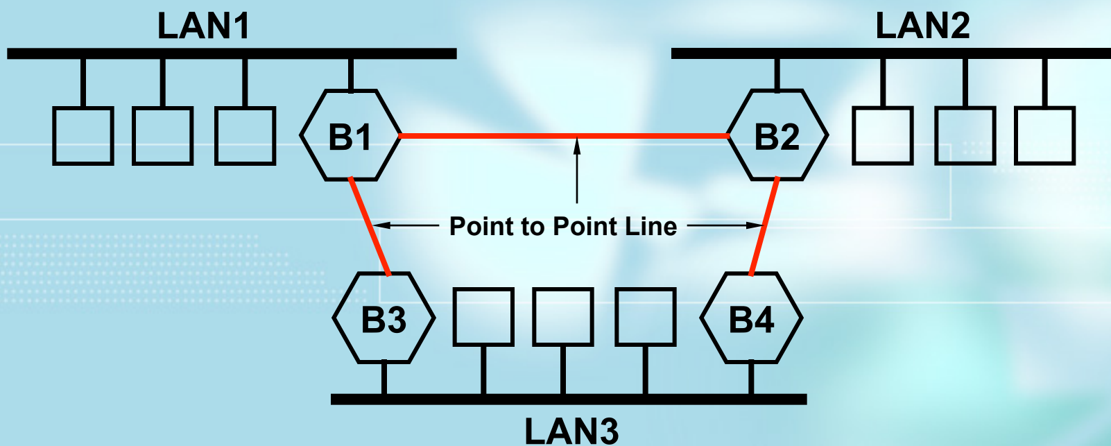
Tnbnm P325 Fig. 4-45 远程网桥连接远距离的LANs
