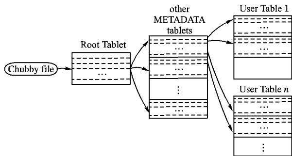
图 3 BigTable 中存储记录板位置信息的结构
