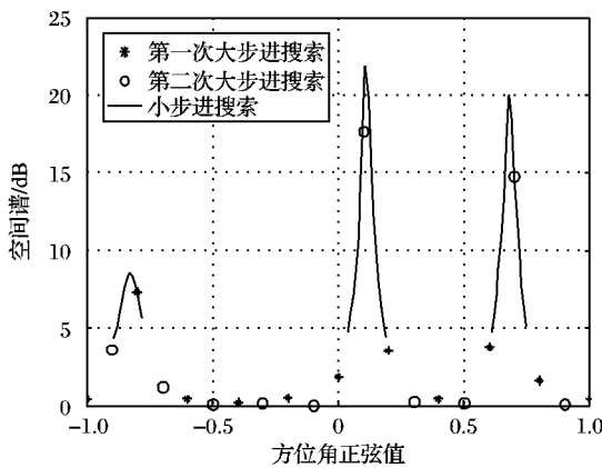
图 2 改进 MUSIC 算法的空间谱
