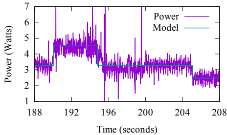
Fig. 5. AT&T Modeling
