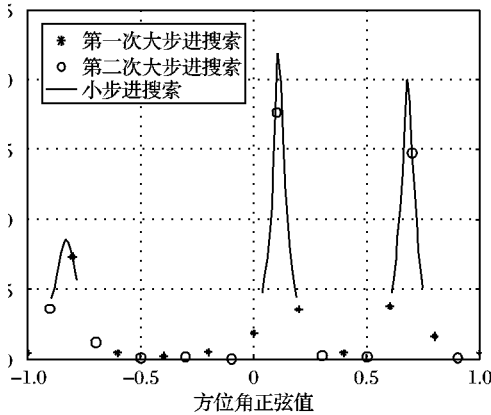
图2 改进 MUSIC 算法的空间谱
